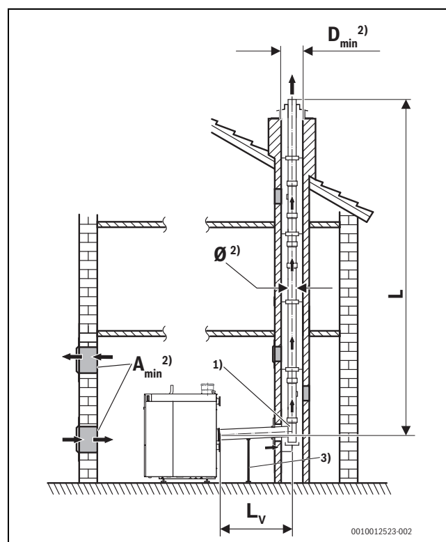
Fig. 18 Évacuation des fumées dans le conduit, variante 1
