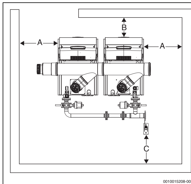
Fig. 9 Distances par rapport aux murs KB372-150...600 – Cascade de 2 chaudières en usine (sans voie d'entretien)
