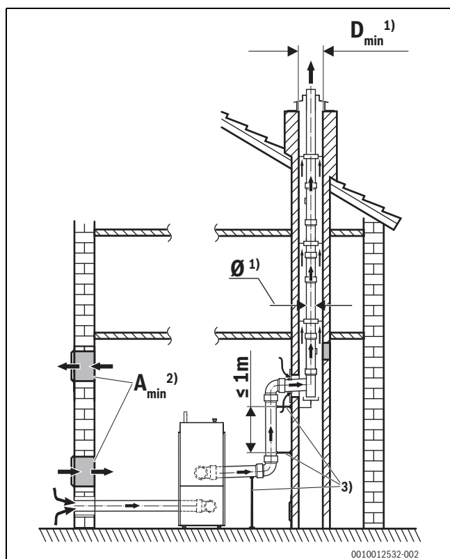
Fig. 24 Tuyaux séparés
