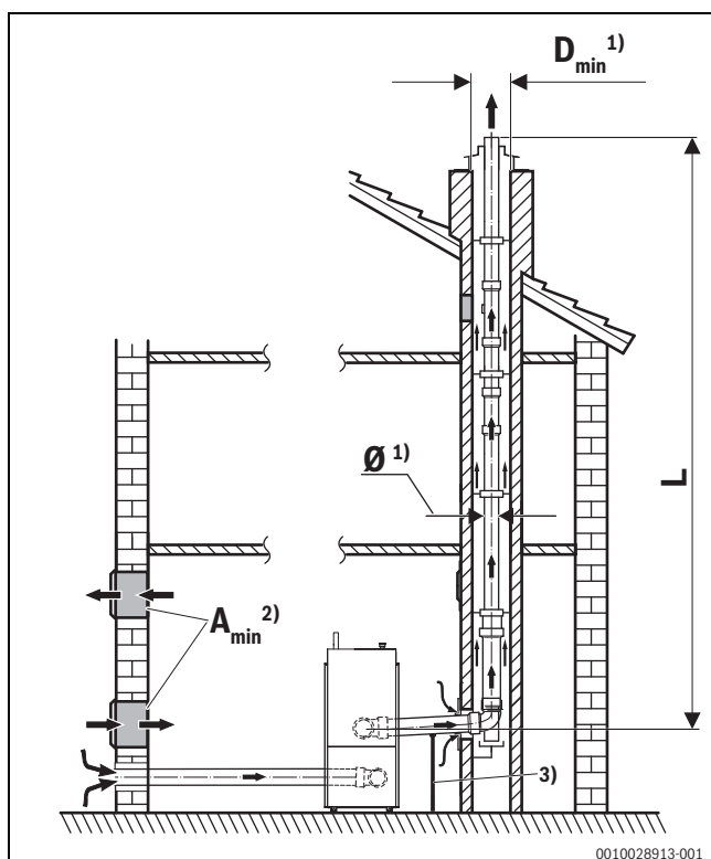
Fig. 26 Hauteur effective de la conduite d'évacuation des fumées, dans le conduit, variante 1
