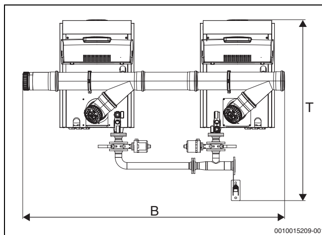
Fig. 10 Cascade de chaudières avec vanne d'isolement et voie d'entretien
