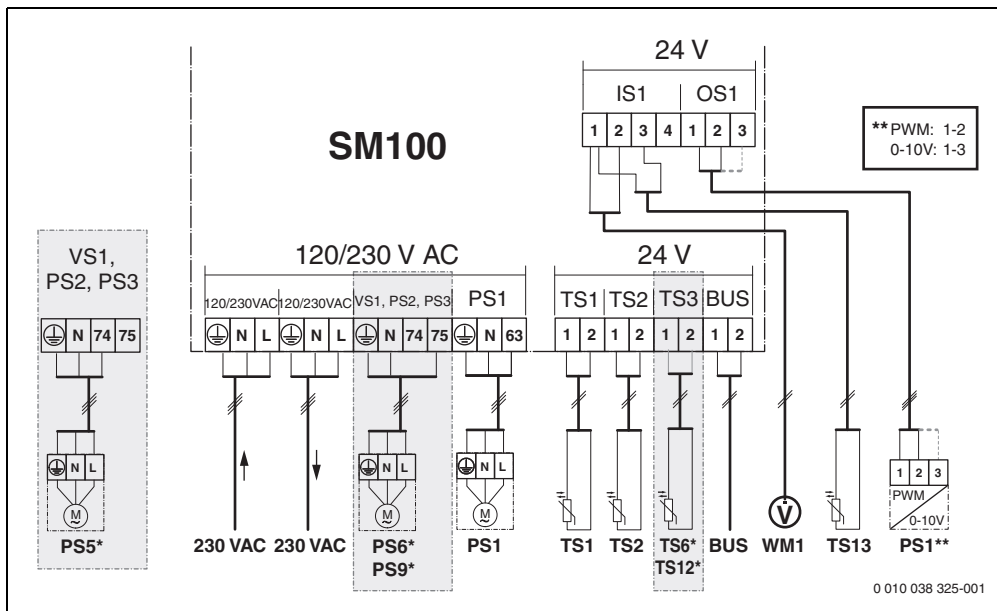
Bild 1 Anschlussklemmenbelegung für Solaranlage
