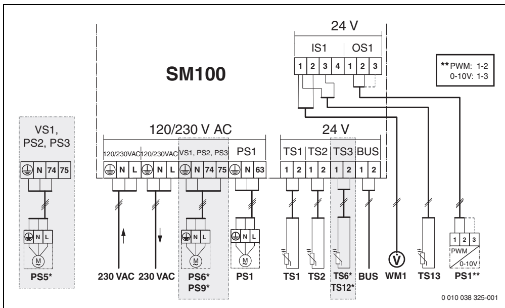
Fig. 1 Morsetti per collegamento del sistema solare termico
