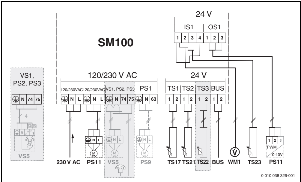
Bild 2 Anschlussklemmenbelegung für Frischwassersystem
