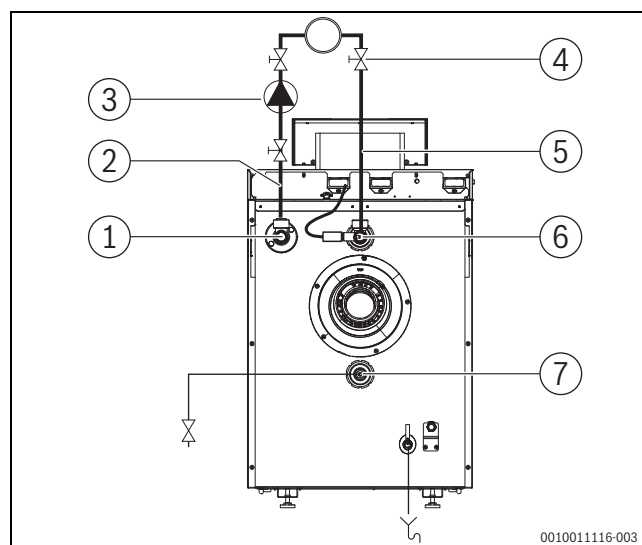
Bild 15 Anschlussschema Hydraulik
