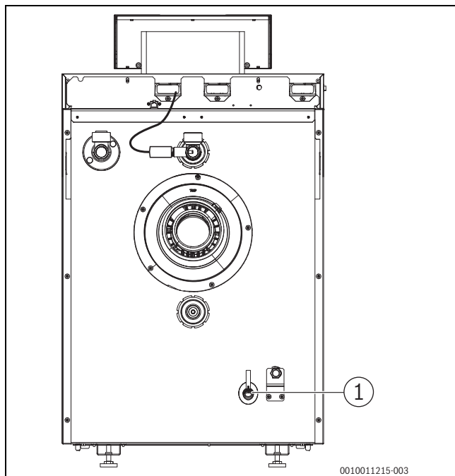
Bild 14 Kondensatschlauch montieren
