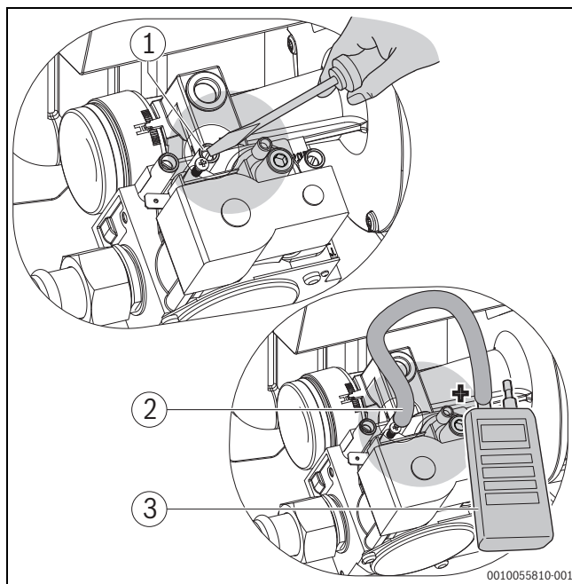
Bild 41 Gas-Luft-Verhältnis kontrollieren und einstellen
