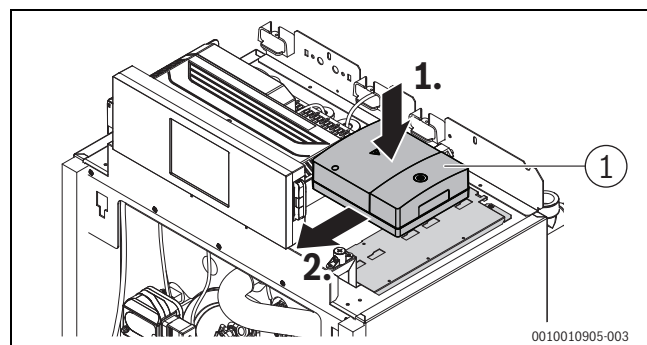
Bild 26 Funktionsmodule einstecken
