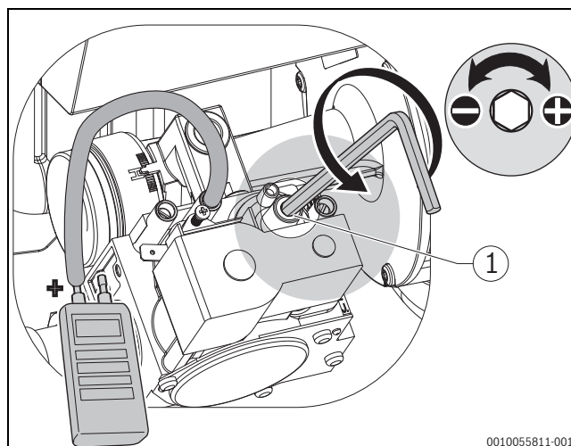
Bild 42 Einstellung Teillast
