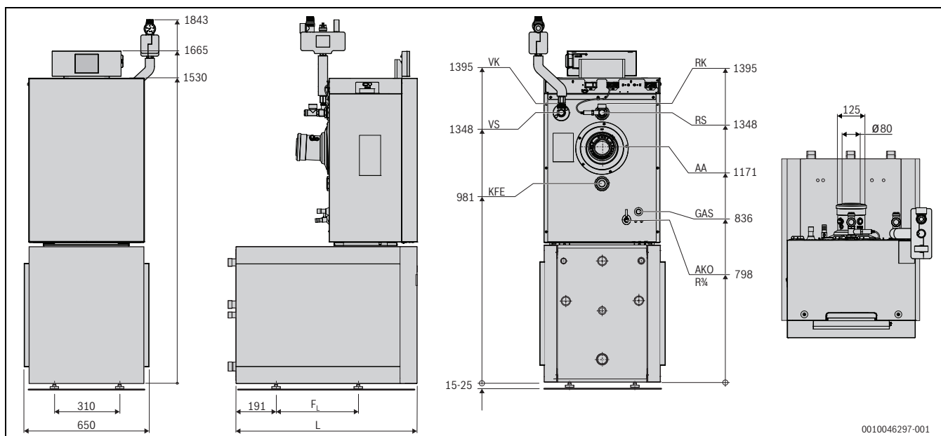
Bild 4 Abmessungen und Anschlüsse Logano plus KB192i.2 mit Logalux L135...L200.3 RS (Maße in mm)
