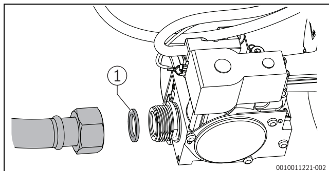
Bild 52 Gasrohr abnehmen
