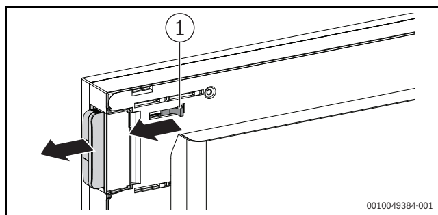
Bild 35 Kommunikationsmodul montieren
