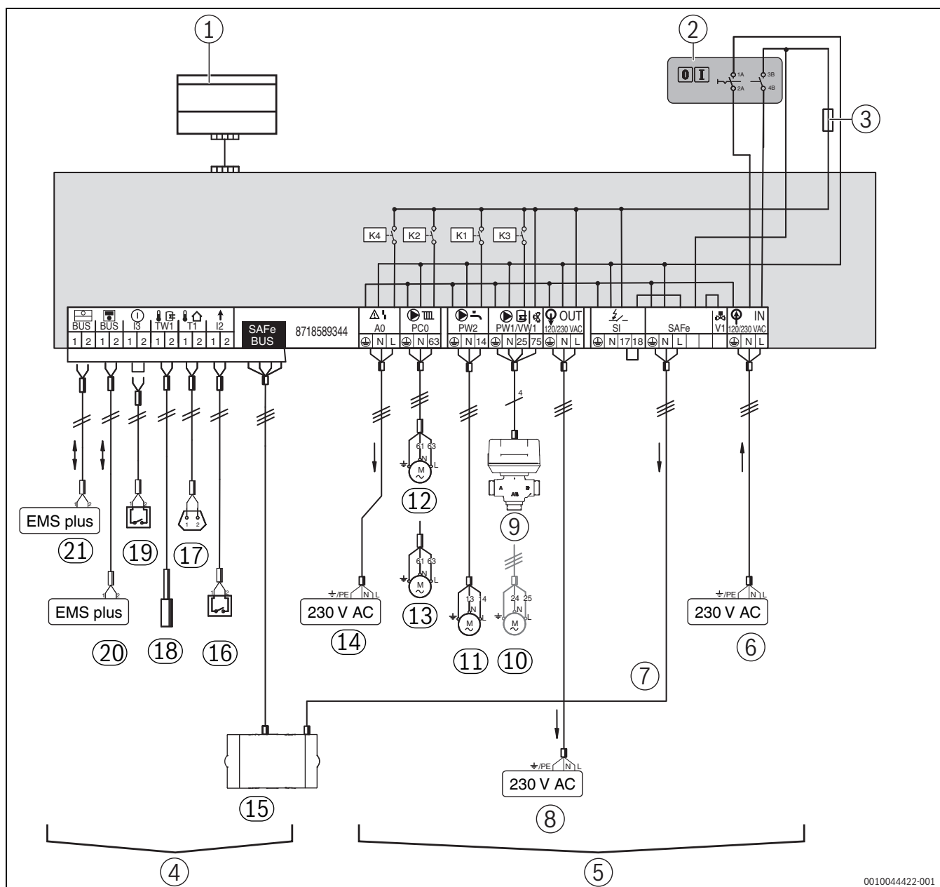
Bild 76 Anschlussplan Regelgerät IMC120
