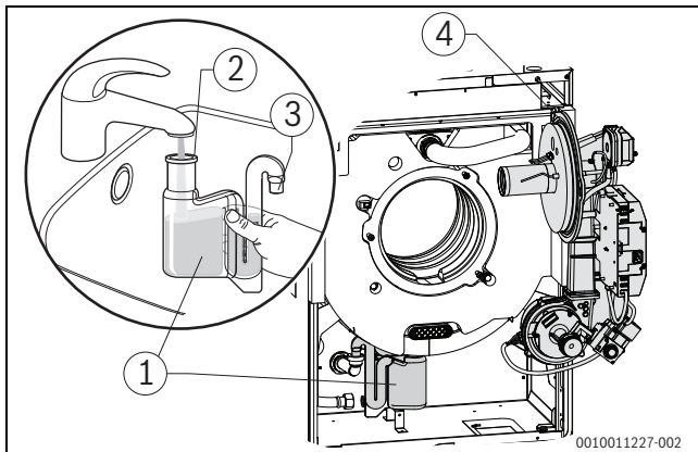
Bild 60 Siphon reinigen
