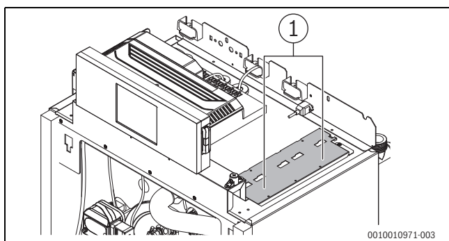
Bild 78 Ansicht ohne Abdeckhaube und ohne Module
