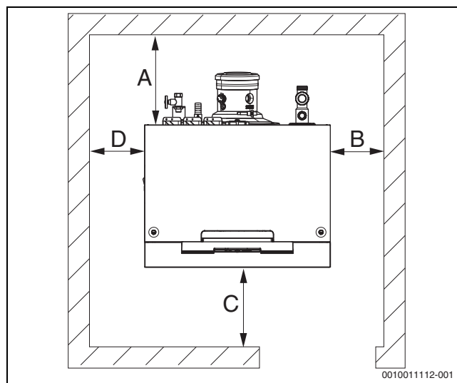
Bild 8 Wandabstände im Aufstellraum
