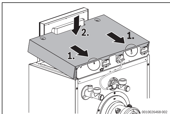
Bild 24 Kesselhaube montieren
