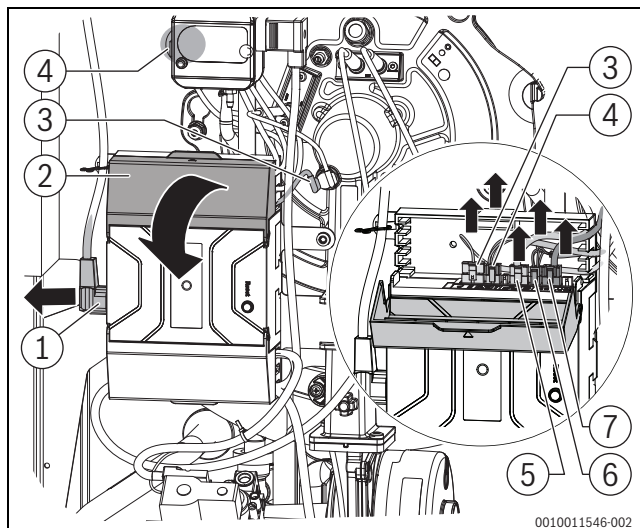
Bild 50 Steckverbinder lösen
