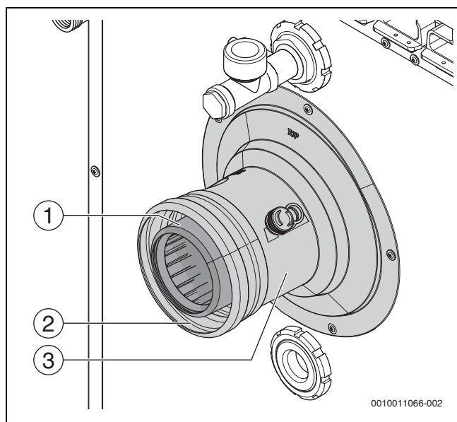
Bild 16 Abgasanschluss montieren
