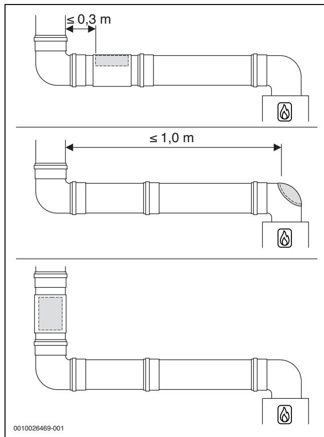
Bild 1 Anordnung der unteren Prüfföffnung
