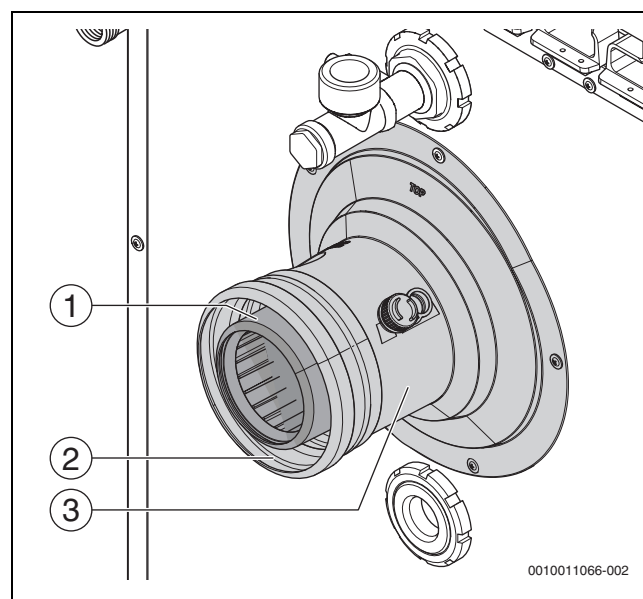
Bild 15 Abgasanschluss montieren
