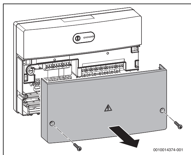
Fig. 13 Retirer le couvercle du module électronique
