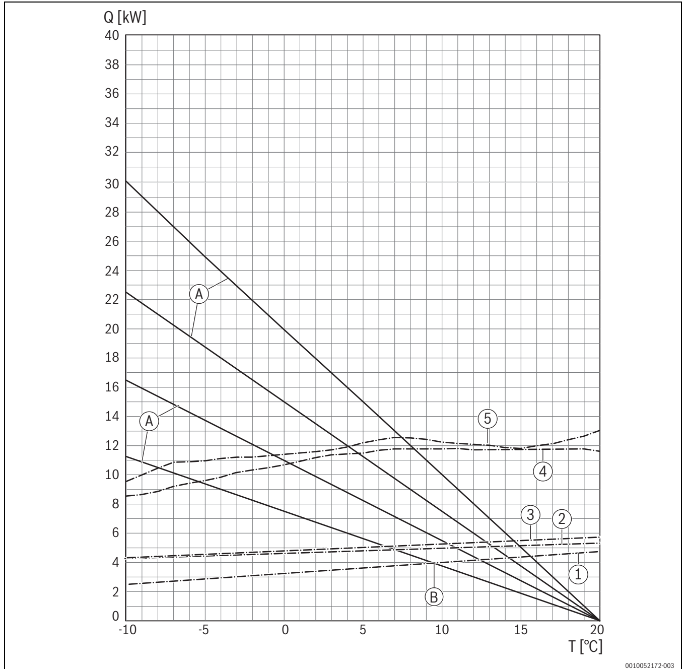
Fig. 24 Diagramme du tableau 9 ; pour déterminer les points de bivalence de la température pour une température de départ de 65 °C
