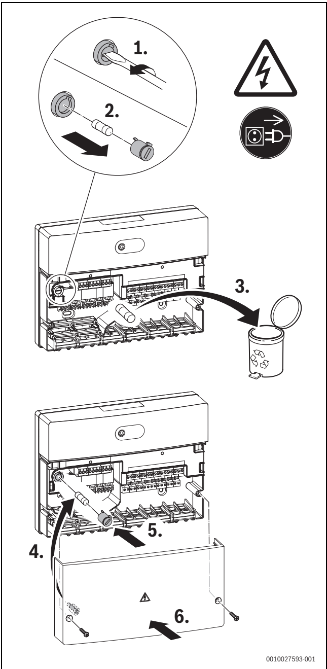
Fig. 27 Remplacer le fusible
